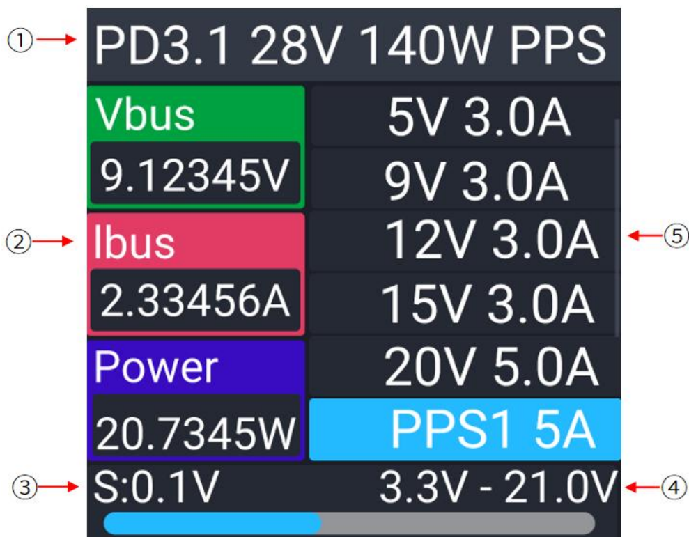
图 2.9 PD 协议手动触发调压 界面
