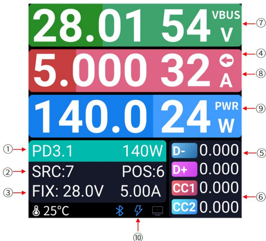
图 2.2 基本测量 界面
