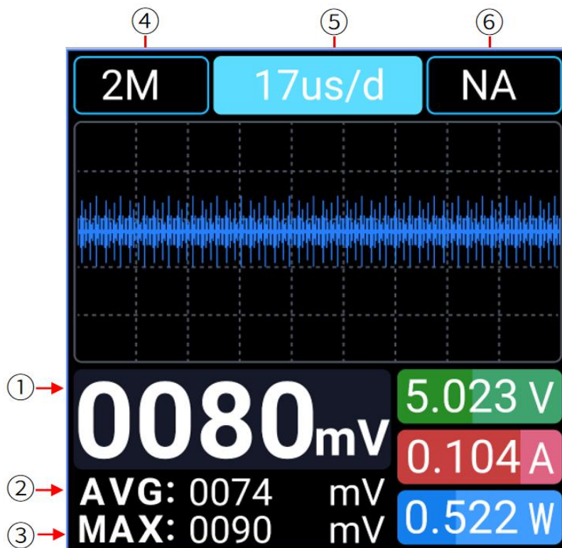
图 2.3 纹波测量界面
