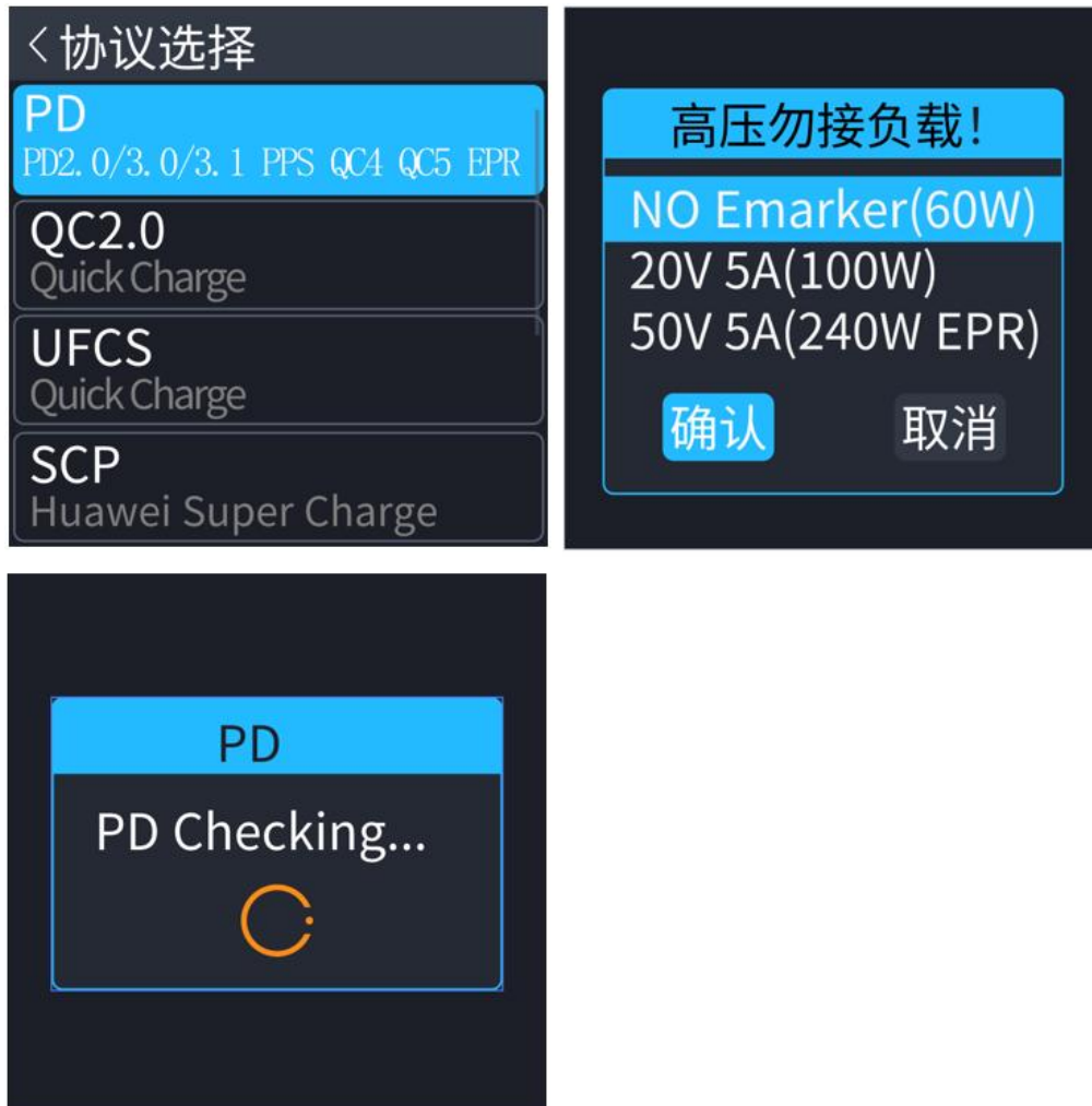
图 2.8 PD 协议手动触发 界面
